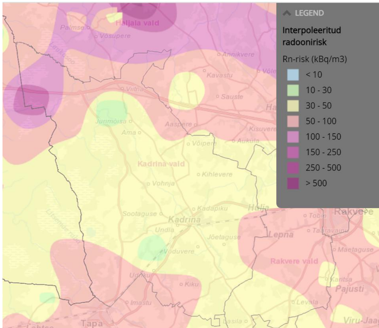
Joonis 6.4 Pinnase interpolateeritud radoonirisk (Allikas: väljavõte Eesti pinnase radooniriski kaardirakendusest, Eesti Geoloogiateenistus, 2021)
