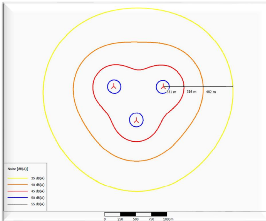
Joonis 14. Illustriativne mürakaart. Modelleeritud on kolmest tuulikust koosnevat tuulikute gruppi tasasel ja takistustevabal maastikul. Tuulikute müraemissiooniks on võetud 108 dB. Tuulikute müra norm elamualadel on 40 dB.
