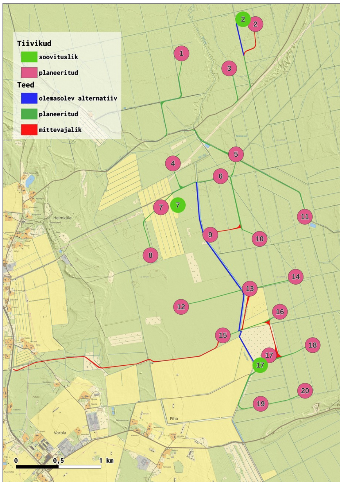
Joonis 6-26 Tuulikute asukohtade ja teedevõrgu optimeerimise soovitused
