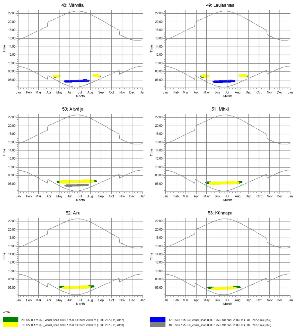
Joonis 6-19 Enim mõjutatud elamupiirkondade varjude esinemise kalender (maksimaalne teoreetiline olukord). Kalendrist on võimalik välja lugeda konkreetses piirkonnas (küll aga ainult päikesepaistelisel ning tuulisel päeval) esineva varjutamise ilmnemise kuupäev ja kellaaeg ning varjutamist põhjustava tuuliku number (erineva värviga on tähistatud erinevatest tuulikute tingitud varjutamine)
