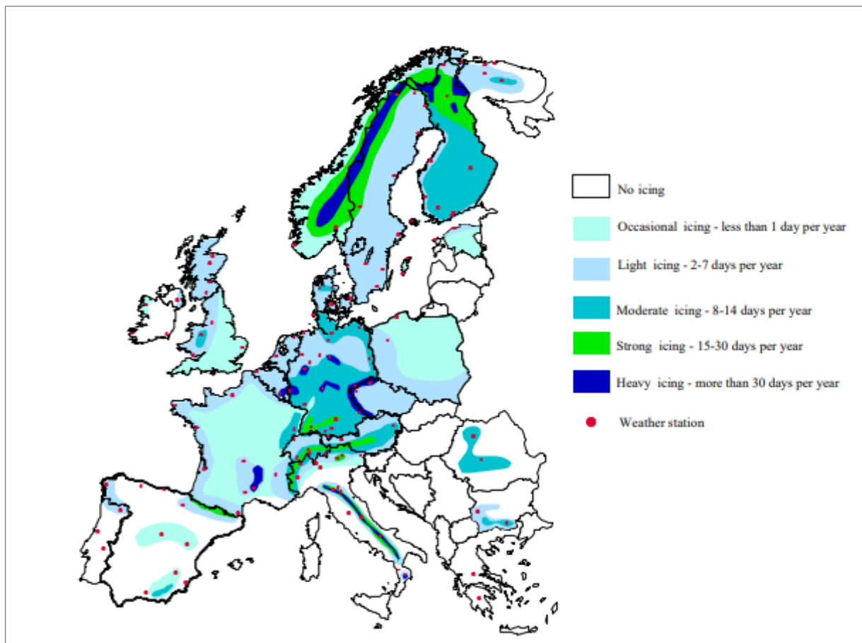
Joonis 6-33 Tuulikute jäätumisohtu käsitlev jääkaart 72
